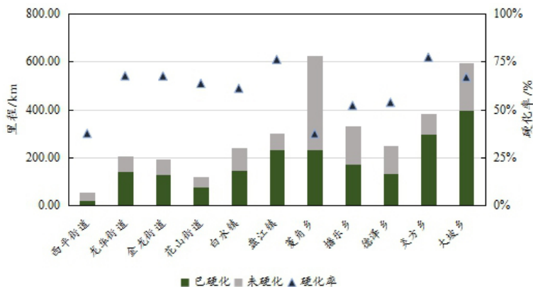
图3.沾益区各乡（镇、街道）农村公路整体硬化情况
